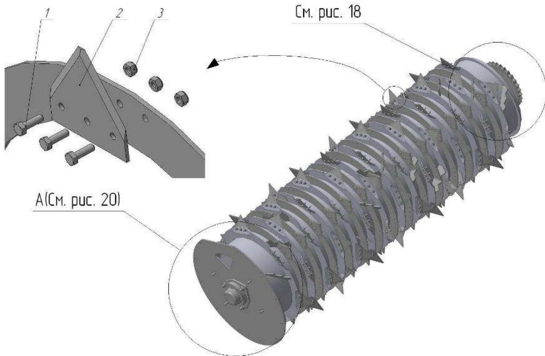
Рисунок 19 – Измельчитель верхний
