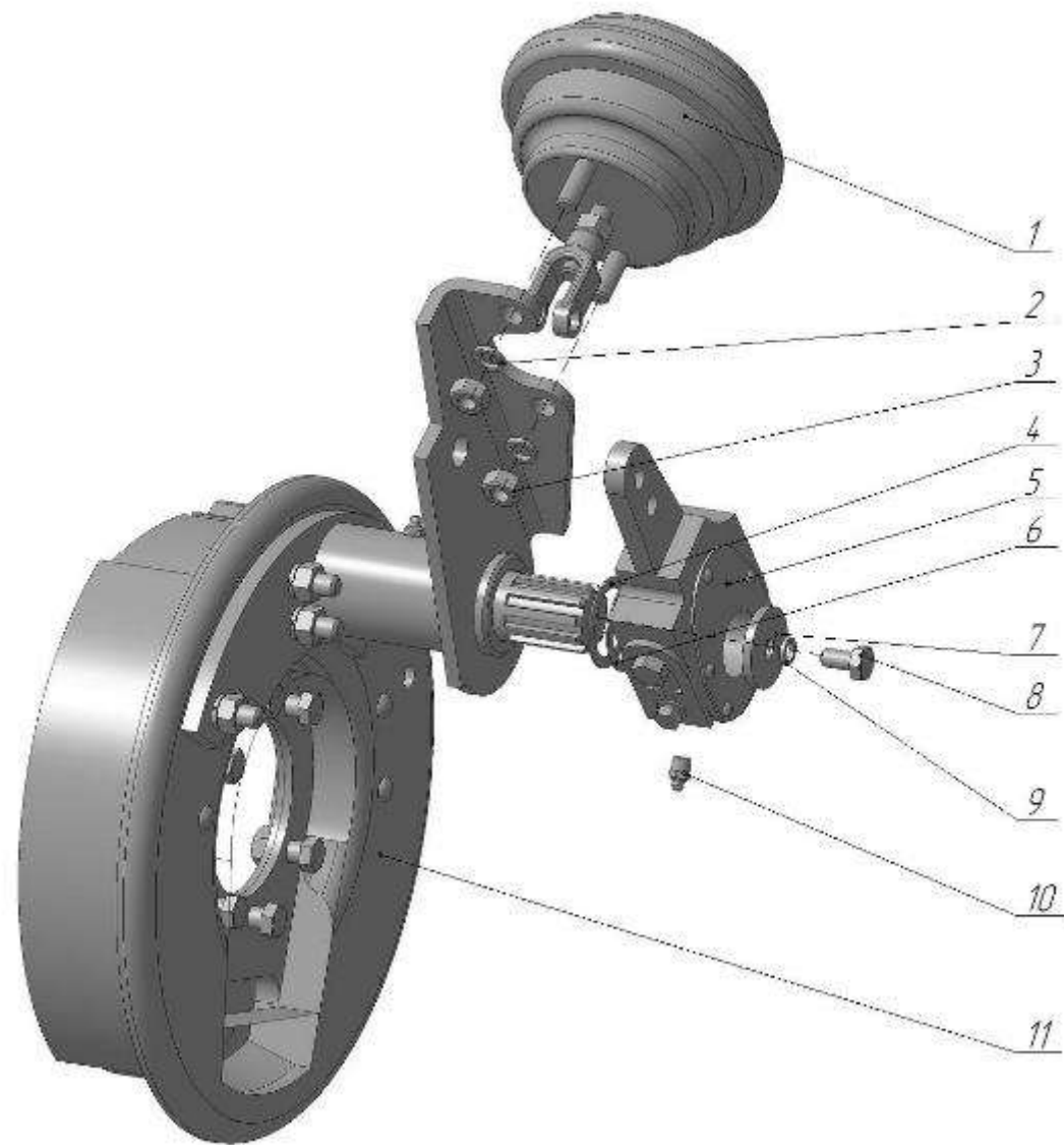
Рисунок 6 – Тормоз в сборе с пневмокамерой
