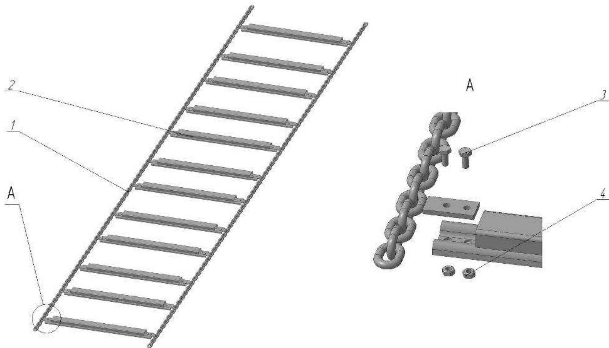
Рисунок 11 – Транспортер
