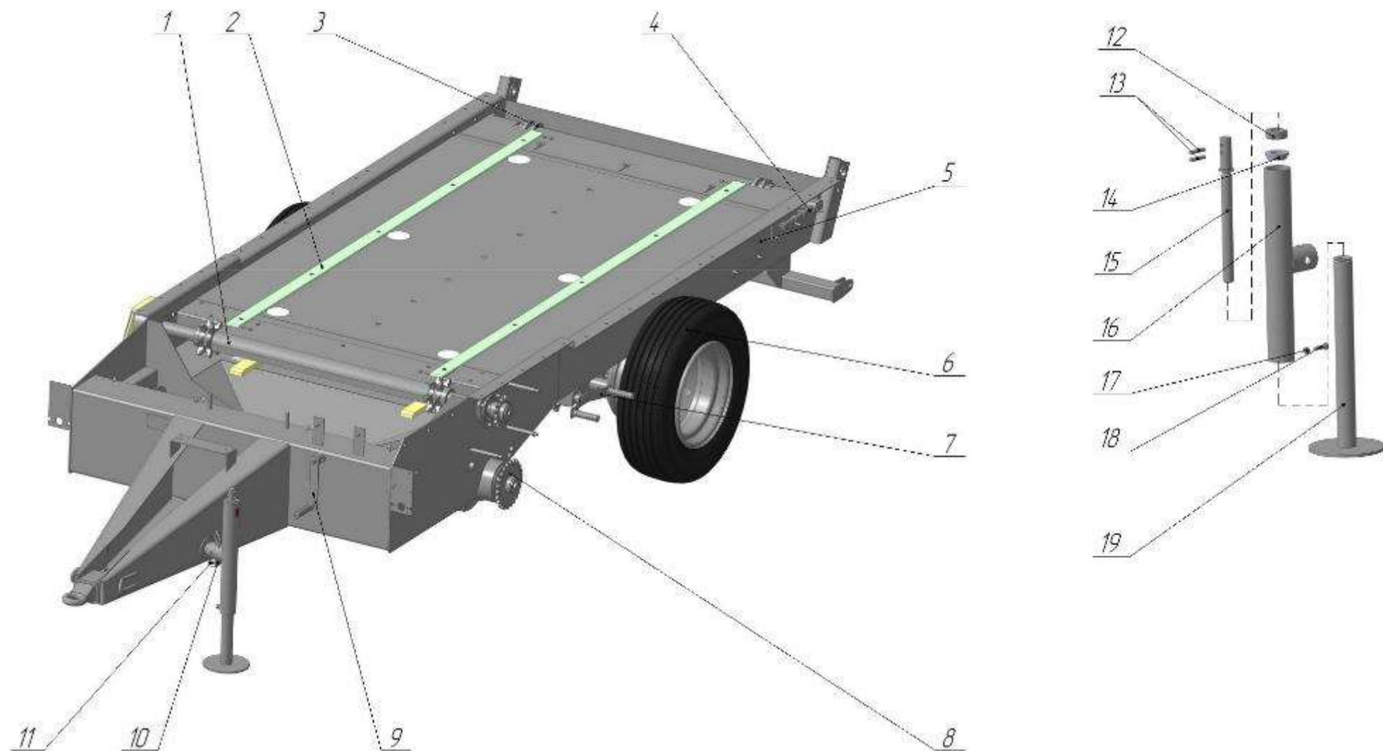
Рисунок 2 – Шасси
