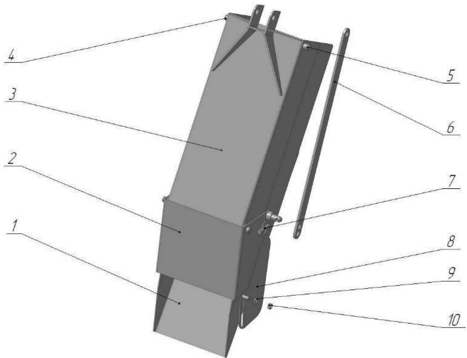
Рисунок 15 – Лоток
