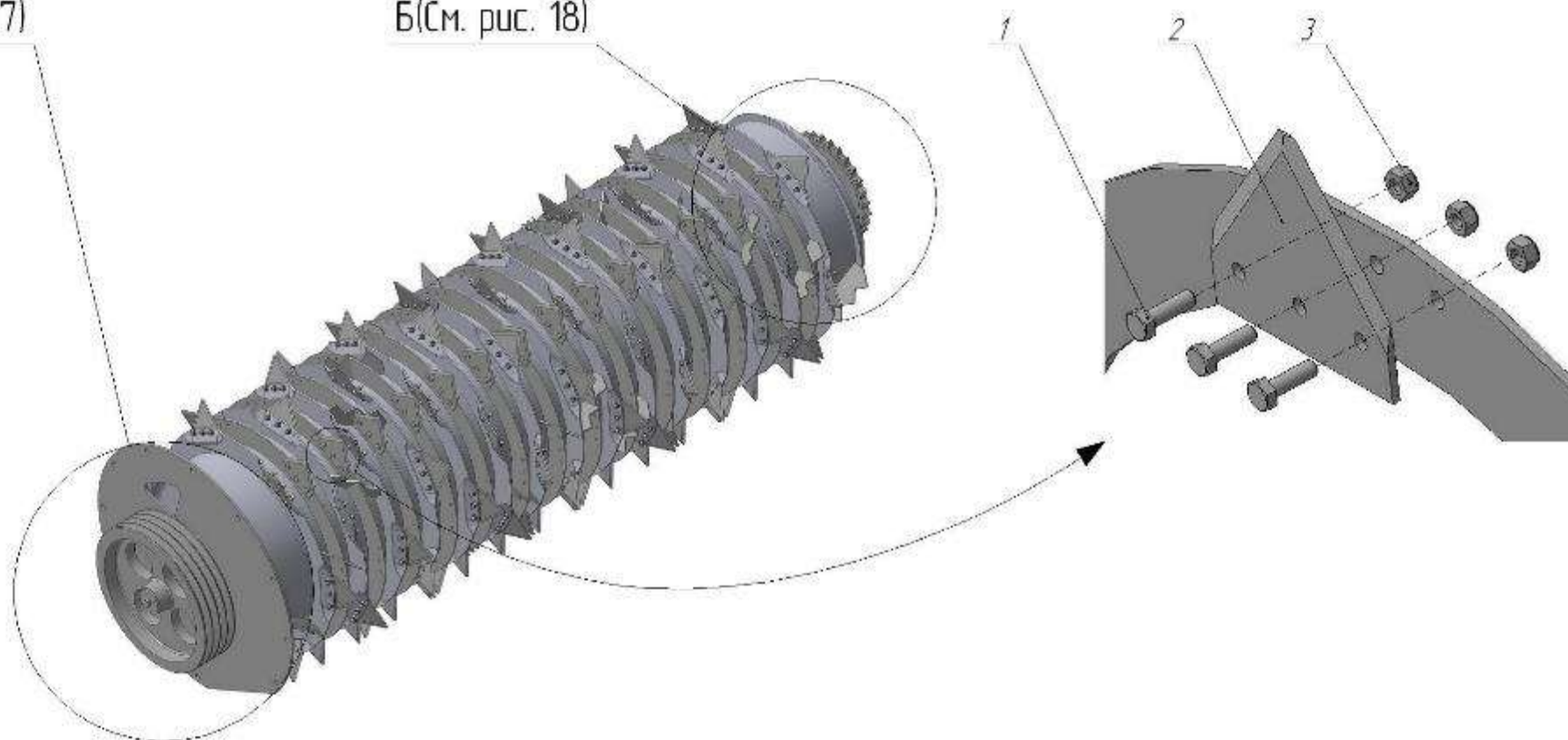
Рисунок 16 – Измельчитель нижний
