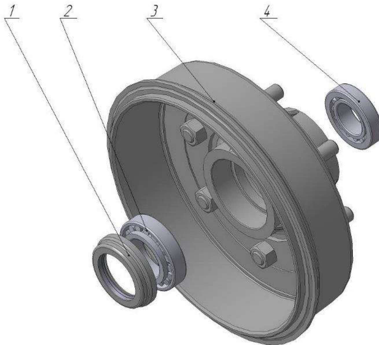
Рисунок 5 – Ступица
