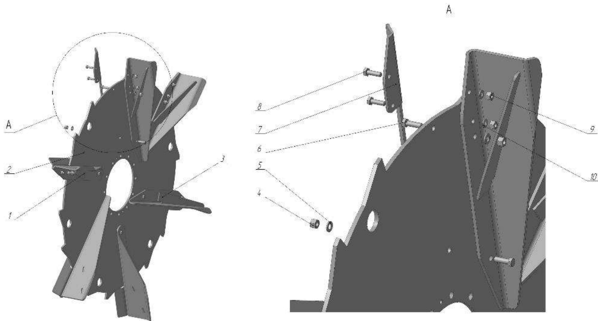
Рисунок 14 – Метатель
