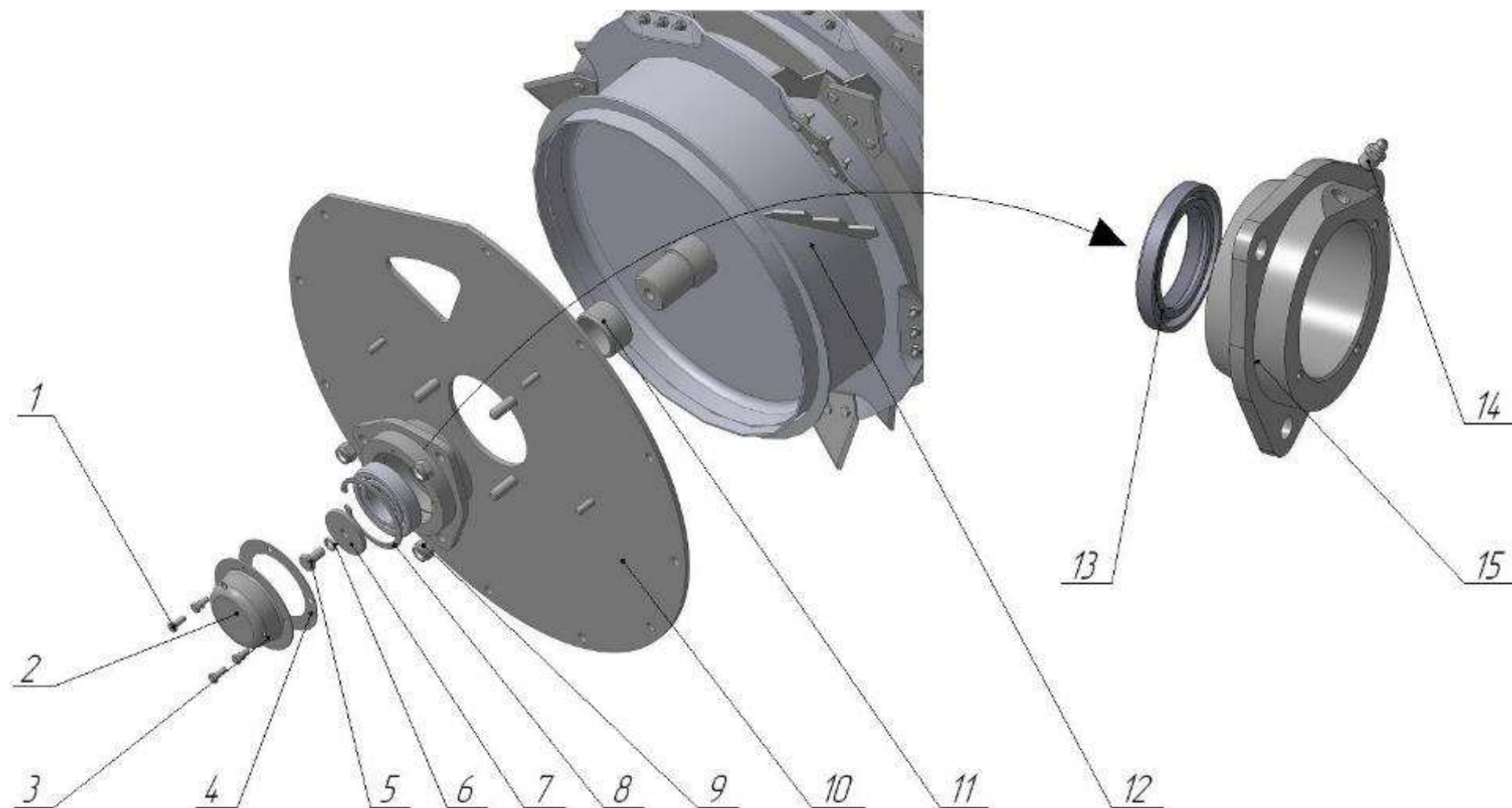
Рисунок 20 – Измельчитель верхний( Вид А)
