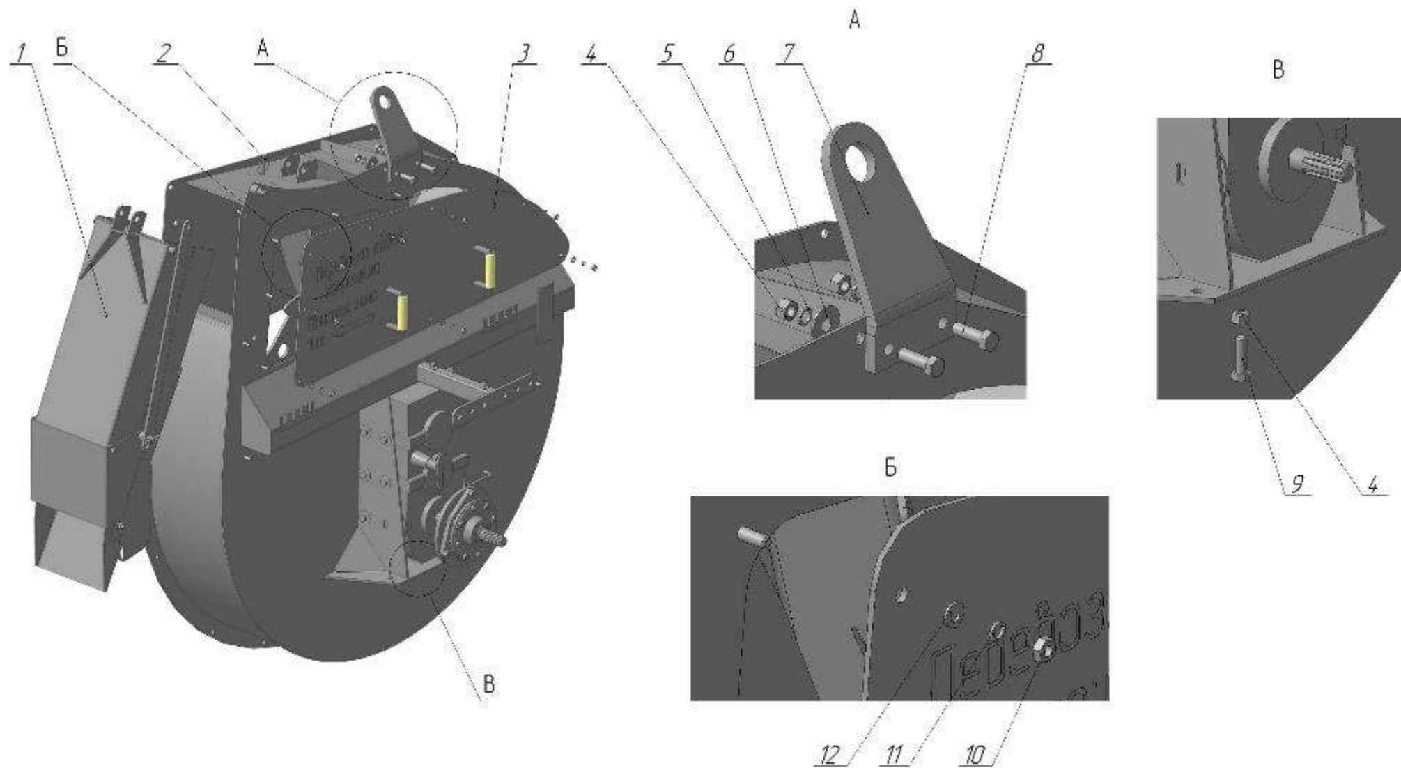
Рисунок 12 – Лобовина
