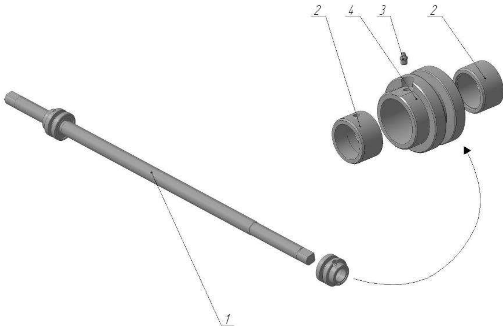
Рисунок 9 – Ось натяжная
