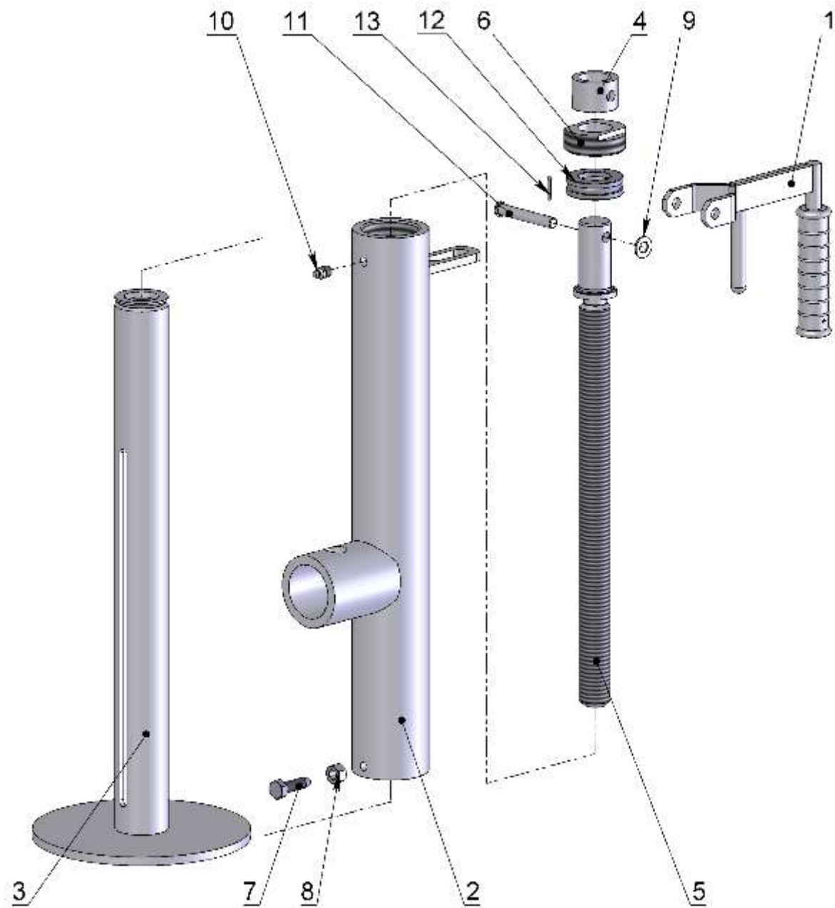
Рисунок 13 – Опора
