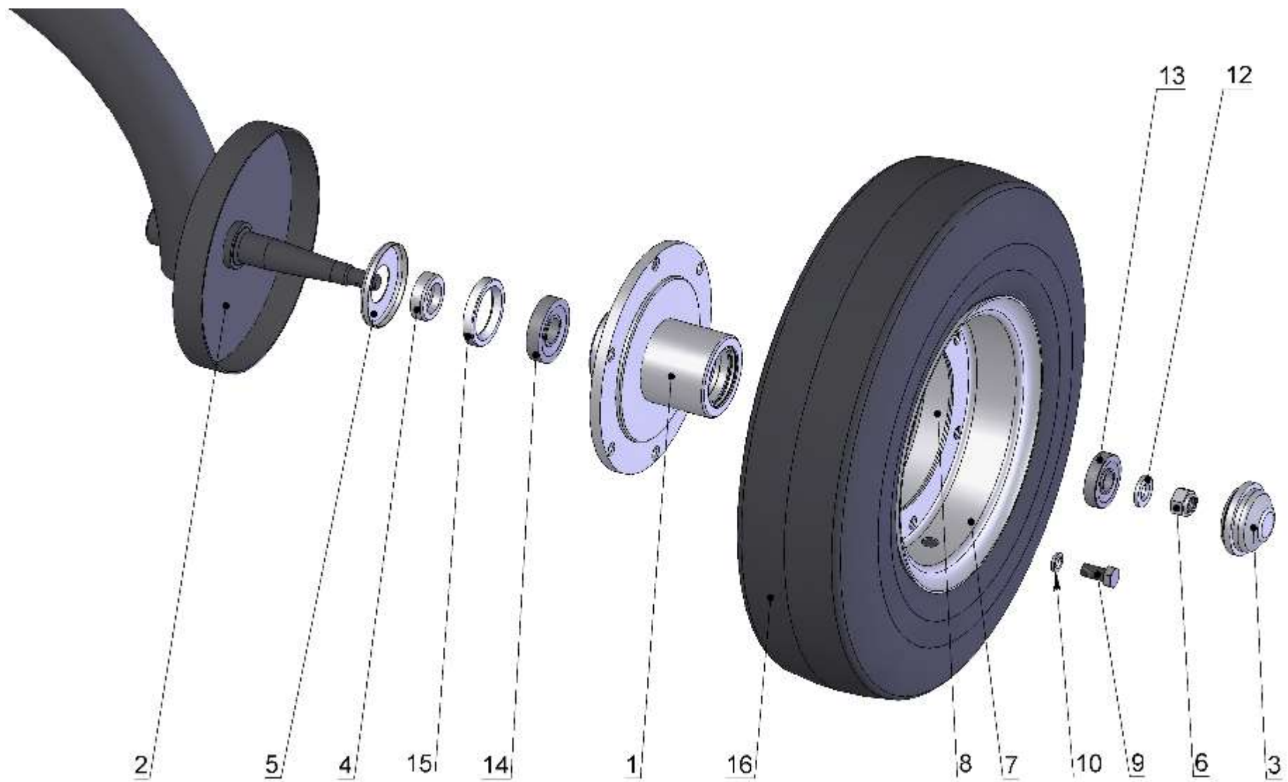
Рисунок 9 – Ход колесный
