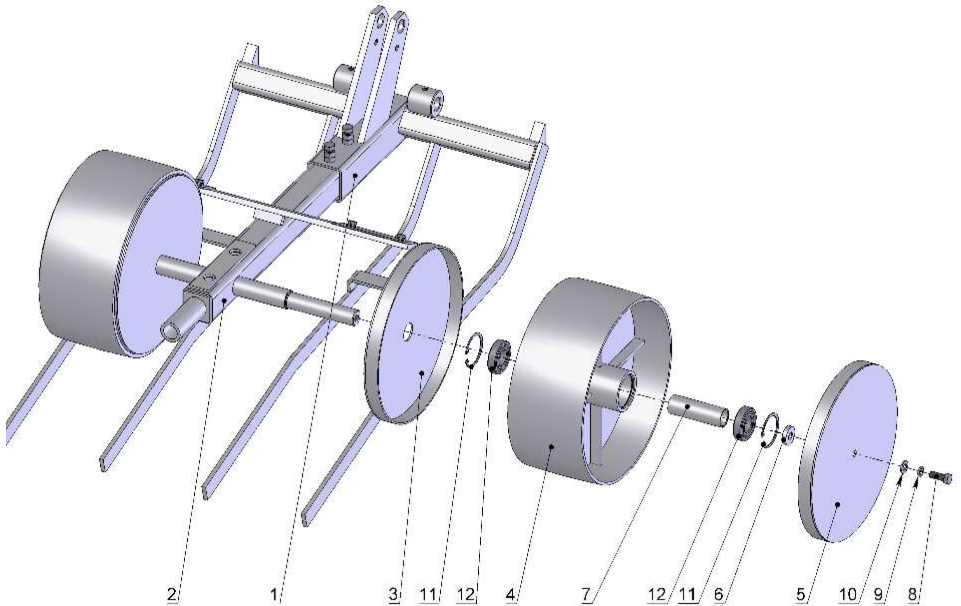
Рисунок 4 – Механизм расстилочный
