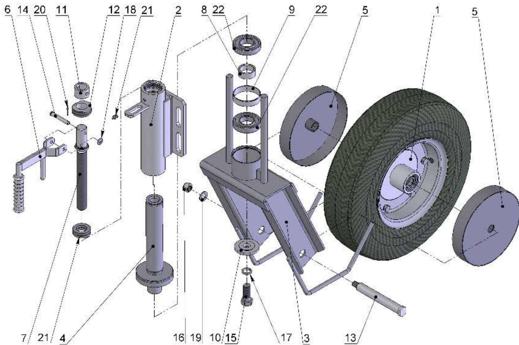
Рисунок 6 – Колесо
