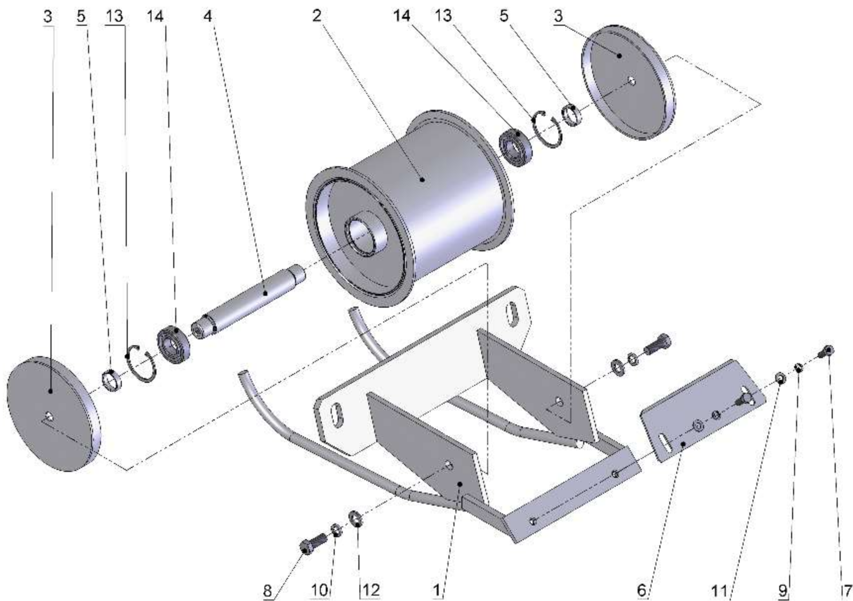
Рисунок 5 – Ролик
