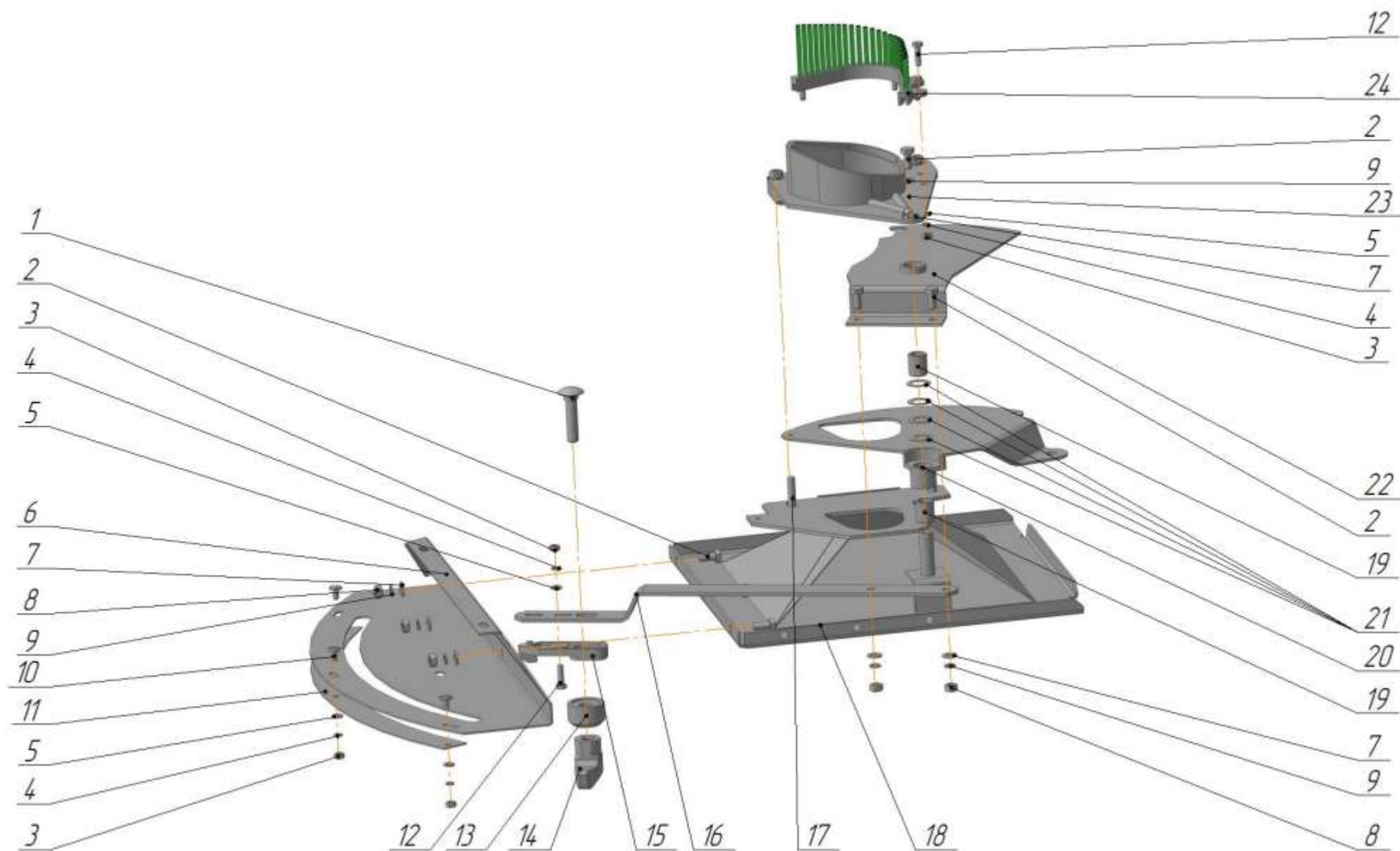
Рисунок 7 – Узел дозирующий
