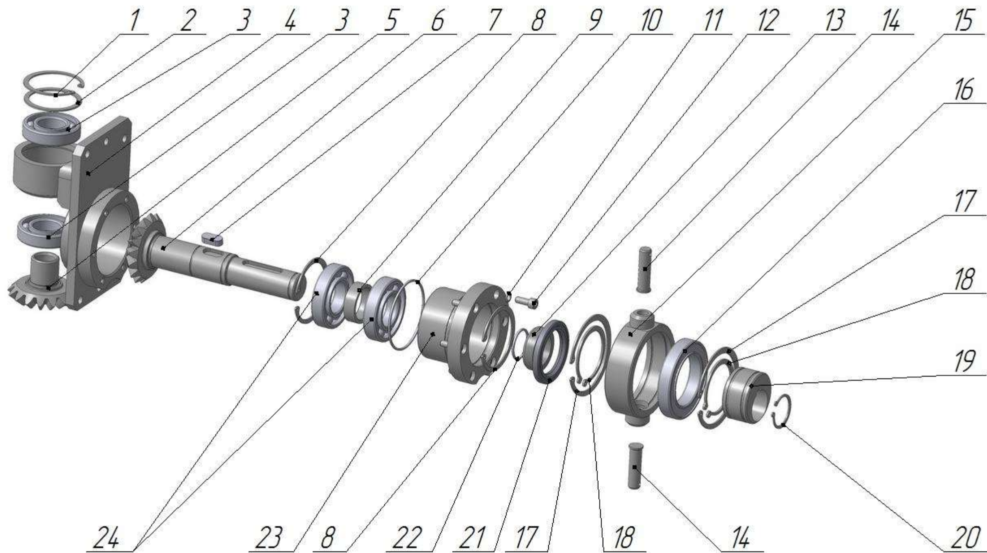
Рисунок 11 – Передача коническая
