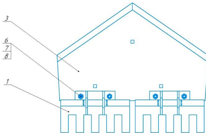
К 19.010-01 СБ Лемех левый
