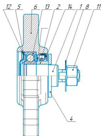
КМ 29.000 Встряхиватель
