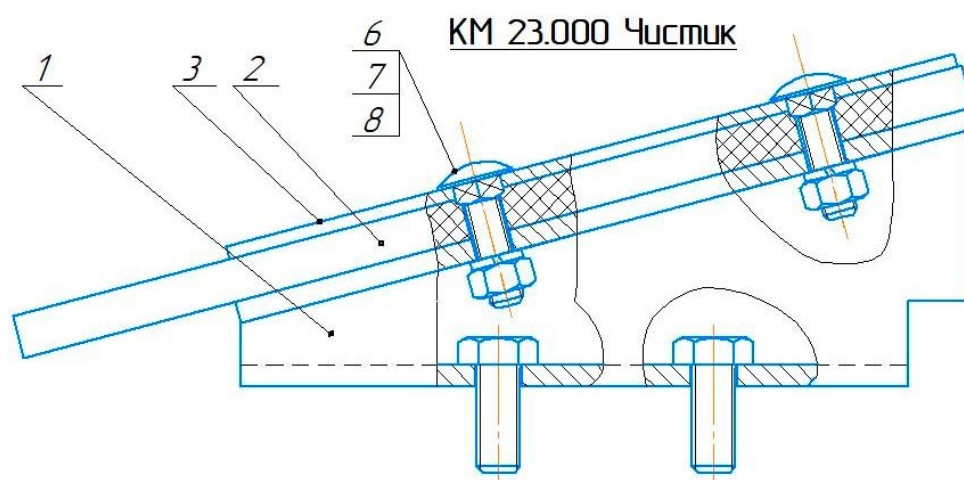
КМ 23.000 Чистик
