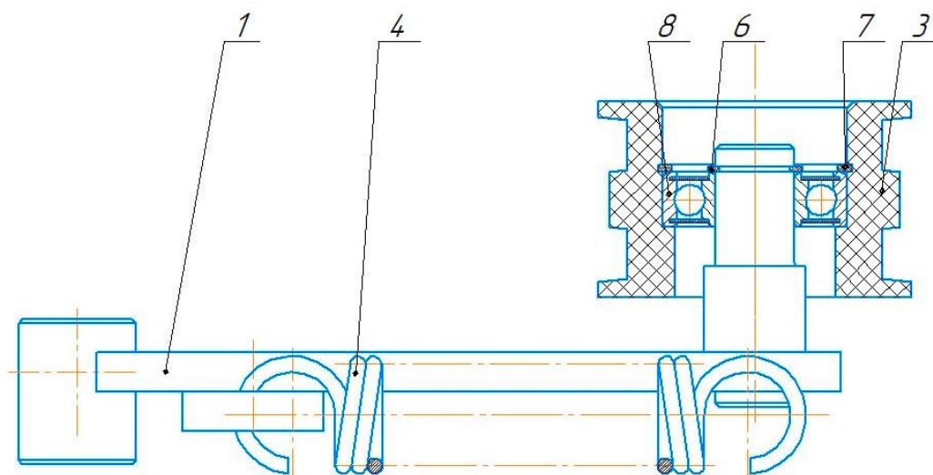
К 35.000 Натяжник
